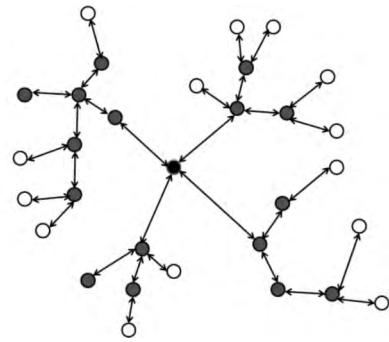
图 2 去掉同层节点间网络链路的 ZigBee 网络
