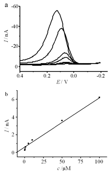
图 7 氧化石墨烯修饰的电极在不同浓度 DA 溶液中的 DPV 曲线(a)及氧化峰电流与 DA 浓度的关系曲线(b)
