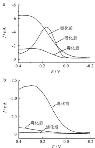
图 5 电极在 100 μmol/L NE(a) 和 1.0 mmol/L AA(b) 溶液中的差分脉曲线
