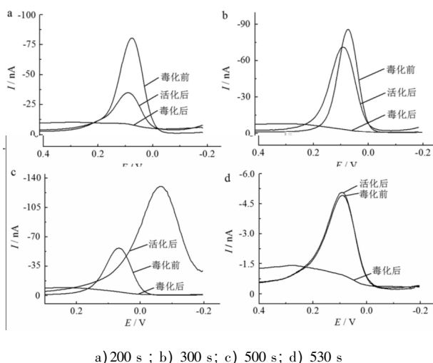
图 3 碳纤维微电极在不同电沉积时间的电化学行为
