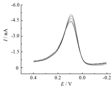
图 4 活化后的电极差分脉冲伏安叠加图
