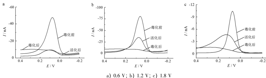
图 2 碳纤维微电极在不同初始电压下的活化效果
