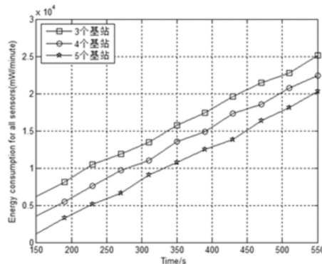
图 2 当基站数分别为 3, 4, 5 时的网络能耗
