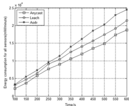
图 3 不同路由算法的网络能耗
